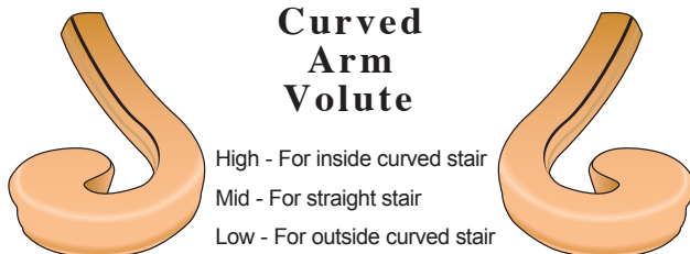
Left Hand 7030CH 7030CM 7030CL
